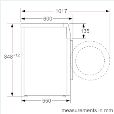
Размерные чертежи
