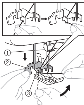
① Игольдержатель ② Рычажок нитевдевателя ③ Направляющая
