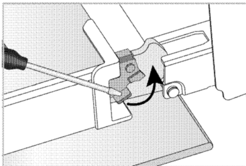
Serratura a cerniera - posizione chiusa
