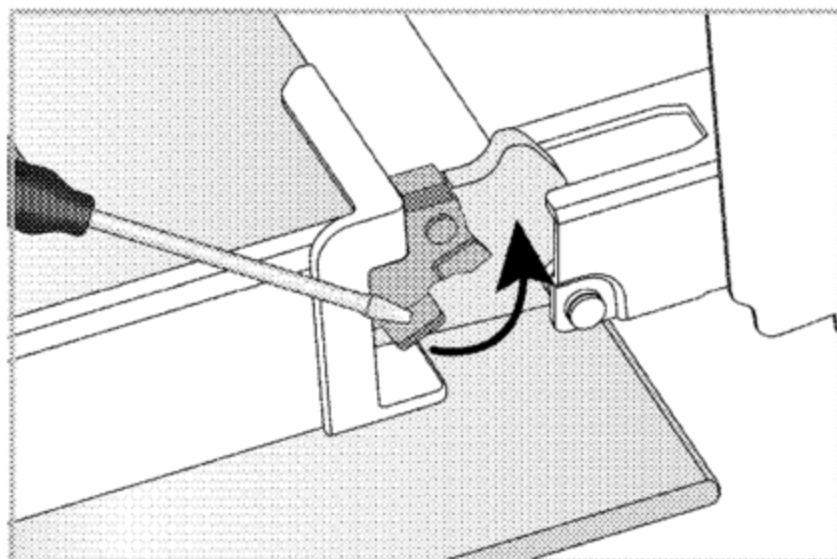
Шарнирный замок - закрытое положение
