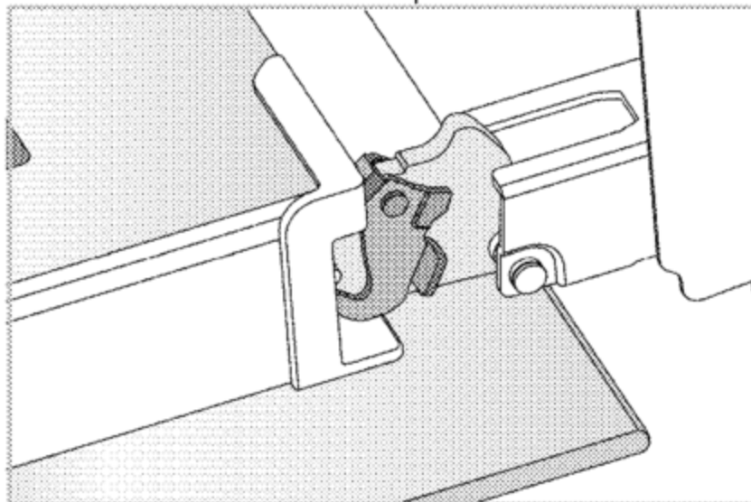
Serratura a cerniera - posizione aperta
